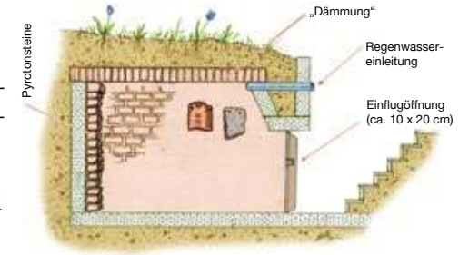
Abb. 47: künstliches Winterquartier
